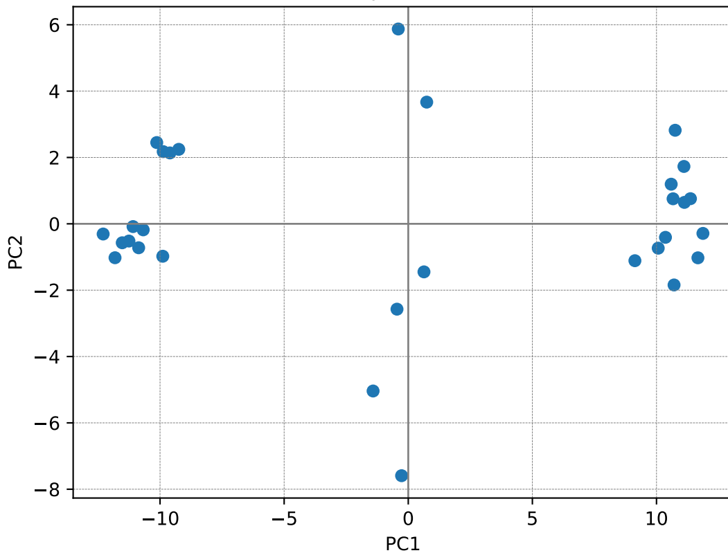
Gráfico de Dispersión: PC1 vs PC2
